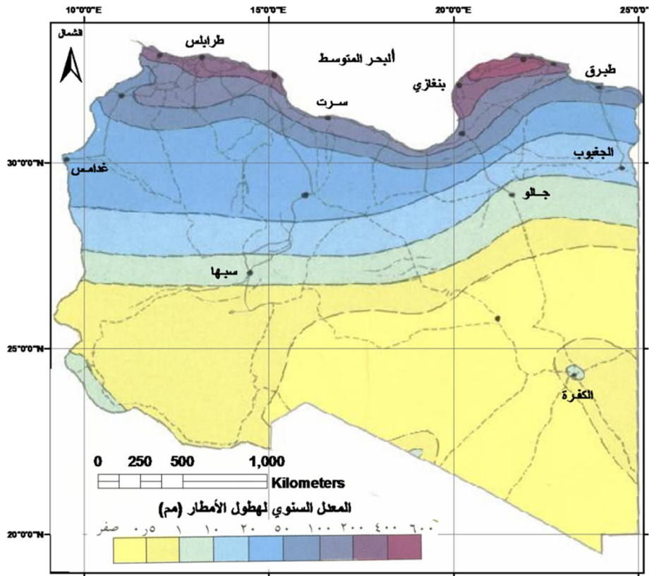
شكل (6.1): المتوسط السنوي لسقوط الأمطار (المصدر: الأطلس الوطني 1978).
